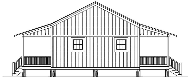
RIGHT ELEVATION
